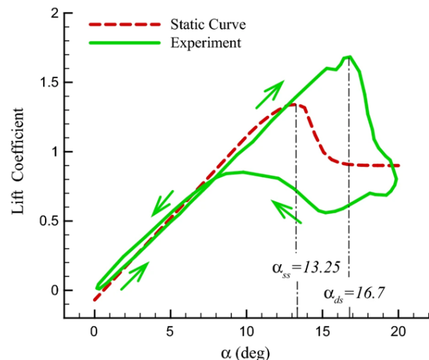
Abbildung 1: Auftriebskoeffizient eines umströmten Profils in Abhängigkeit des zeitlich veränderlichen Anströmwinkels mit statischem Ablösewinkel \alpha_{ss} und dynamischen Ablösewinkel \alpha_{ds} [1]
